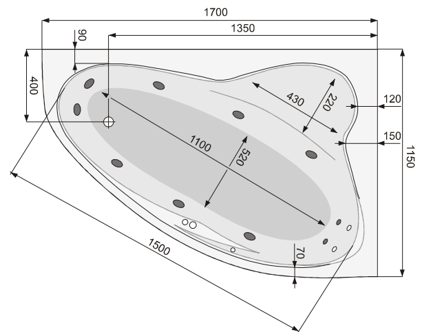
Version rechts
